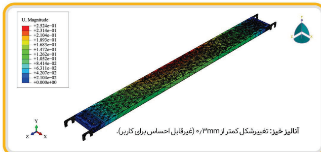
توزیع تنش (Class 4): سطح آبی نشان‌دهنده تنش بسیار پایین و ایمنی بالاست.
