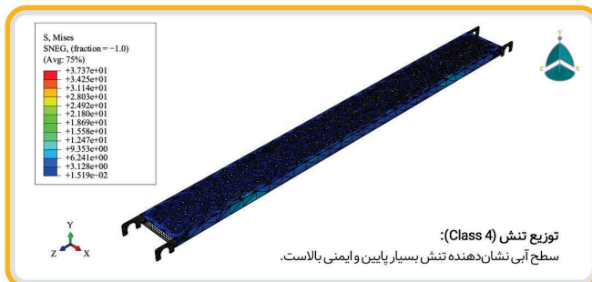
مدل سه بعدی: طراحی بهینه پروفیل و موقعیت استراتژیک تقویت‌کننده‌ها (Stiffeners).
